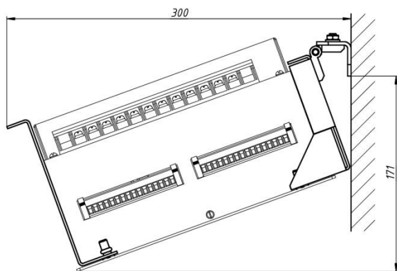
«Орион-2-Х» в положении для подключения проводов к клеммникам аналоговых входов ТТ и ТН
