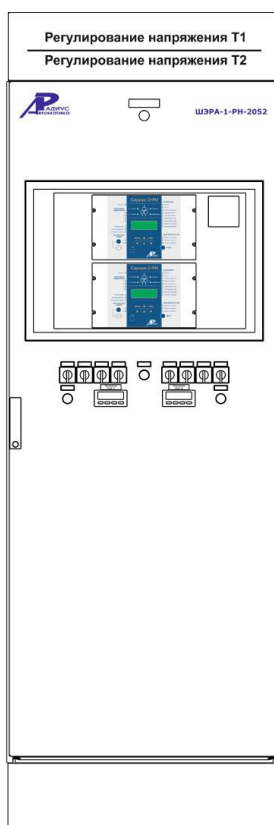
Шкаф регулирования напряжения трансформаторов ШЭРА-1-РН-2052 (БПВА.656457.149, БПВА.650645.001 ТУ)
