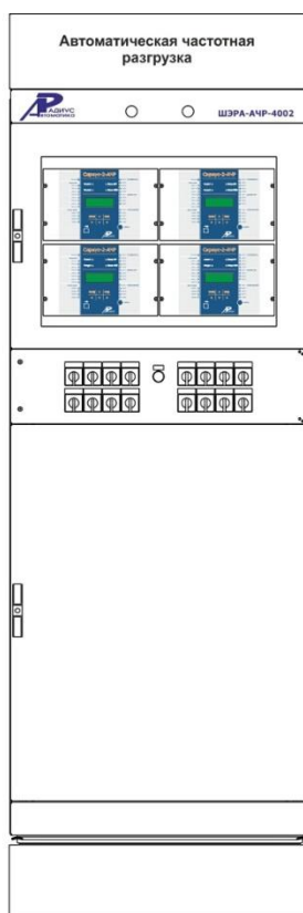
Шкаф автоматической частотной разгрузки ШЭРА-АЧР-4002 БПВА.656457.271, БПВА.650645.001 ТУ
