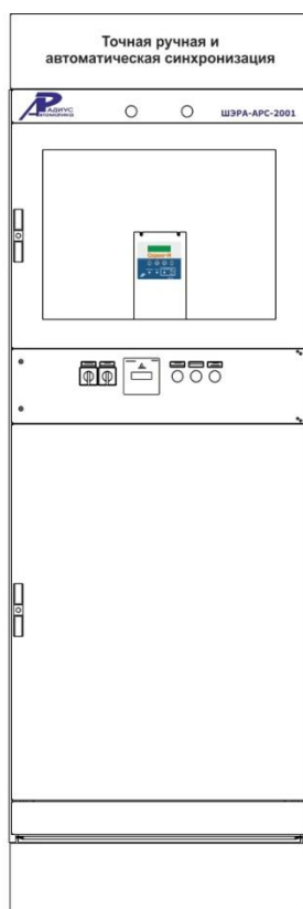
Шкаф точной ручной и автоматической синхронизации ШЭРА-АРС-2001 БПВА.656457.248, БПВА.650645.001 ТУ
