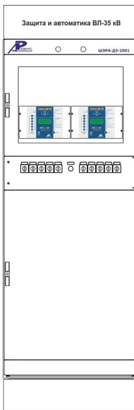
Шкаф дистанционных защит и АУВ линий 6 -35 кВ ШЭРА-ДЗ-2001 БПВА.656457.449, БПВА.650645.001 ТУ
