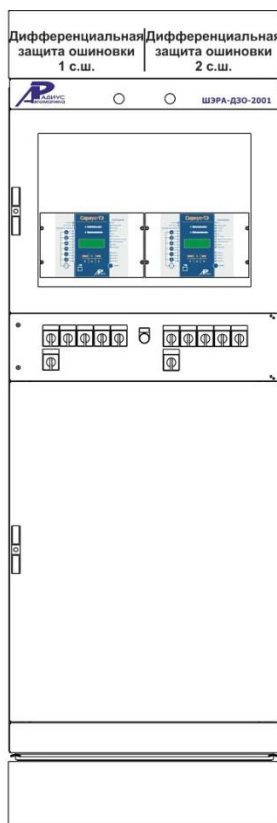
Шкаф дифференциальной защиты ошиновки 110 (220) кВ (до 6 присоединений) ШЭРА-ДЗО-2001 (БПВА.656457.035, БПВА.650645.001 ТУ)
