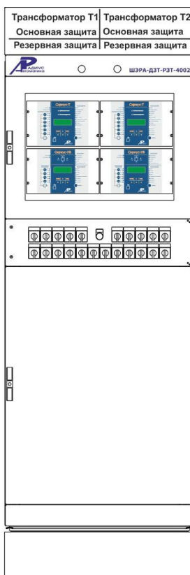
Шкаф основных и резервных защит двухобмоточного трансформатора ШЭРА-ДЗТ-РЗТ-4002 БПВА.656457.444, БПВА.650645.001 ТУ
