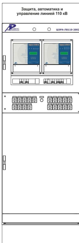
Шкаф защит и АУВ линии 110(220) кВ ШЭРА-ЛВ110-2002 БПВА.656457.081, БПВА.650645.001 ТУ
