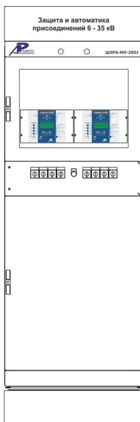
Шкаф защиты и АУВ линий 6-35 кВ (для 2-х линий) ШЭРА-МЛ-2001 БПВА.656457.502, БПВА.650645.001 ТУ
