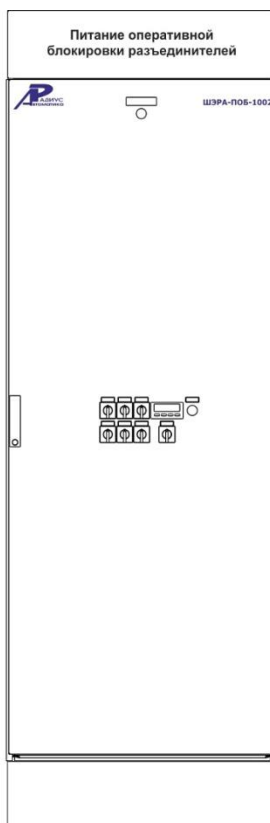
Шкаф питания цепей оперативной блокировки ШЭРА-ПОБ-1002 БПВА.656457.294, БПВА.650645.001 ТУ
