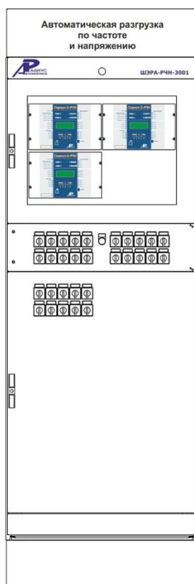
Шкаф автоматического ограничения снижения частоты и напряжения ШЭРА-РЧН-3001 БПВА.656457.220, БПВА.650645.001 ТУ
