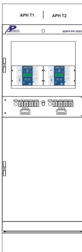
Шкаф регулирования напряжения двух трансформаторов ШЭРА-РН-2053 БПВА.656457.185, БПВА.650645.001 ТУ
