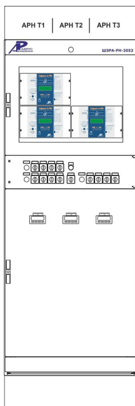
Шкаф регулирования напряжения трех трансформаторов ШЭРА-РН-3053 БПВА.656457.386, БПВА.650645.001 ТУ
