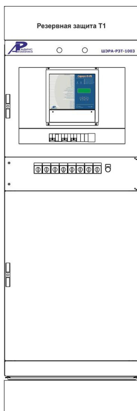
Шкаф резервных защит и АУВ ст. ВН трансформатора ШЭРА-РЗТ-1003 БПВА.656457.510, БПВА.650645. ТУ
