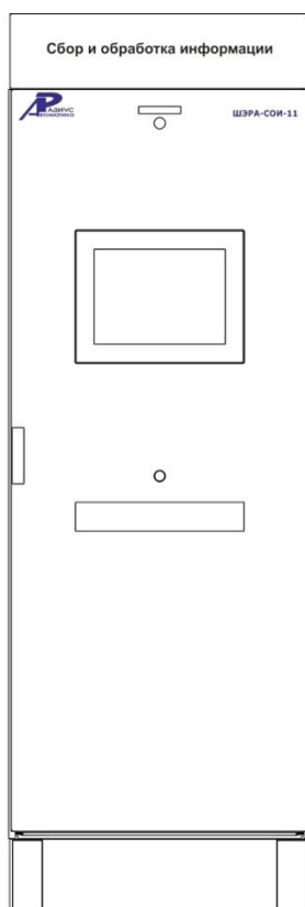
Шкаф сбора и обработки информации (до 32 терминалов) ШЭРА-СОИ-11 БПВА.656457.171, БПВА.650645.001 ТУ
