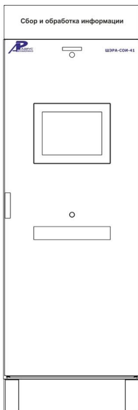
Шкаф сбора и обработки информации (до 128 терминалов) ШЭРА-СОИ-41 БПВА.656457.174, БПВА.650645.001 ТУ
