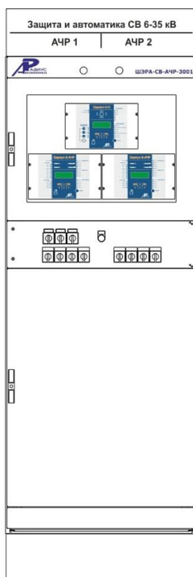
Шкаф защиты и автоматики секционного выключателя 6-35 кВ и АЧР ШЭРА-СВ-АЧР-3001 БПВА.656457.487, БПВА.650645.001 ТУ
