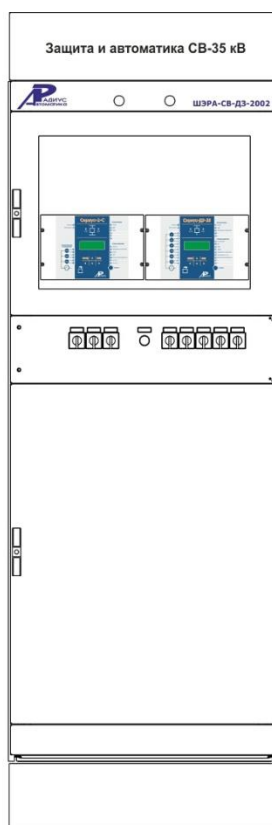
Шкаф защиты и автоматики секционного выключателя и линии 6-35 кВ ШЭРА-СВ-ДЗ-2002 БПВА.656457.450, БПВА.650645.001 ТУ
