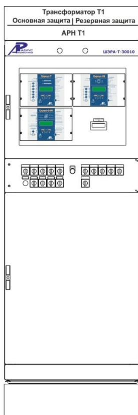
Шкаф защит двухобмоточного трансформатора, АУВ сторон ВН и НН ШЭРА-Т-30010 (БПВА.656457.456, БПВА.650645.001 ТУ)
