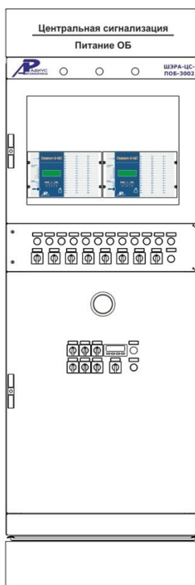
Шкаф центральной сигнализации и питания цепей ОБР ШЭРА-ЦС-ПОБ-3002 БПВА.656457.280, БПВА.650645.001 ТУ
