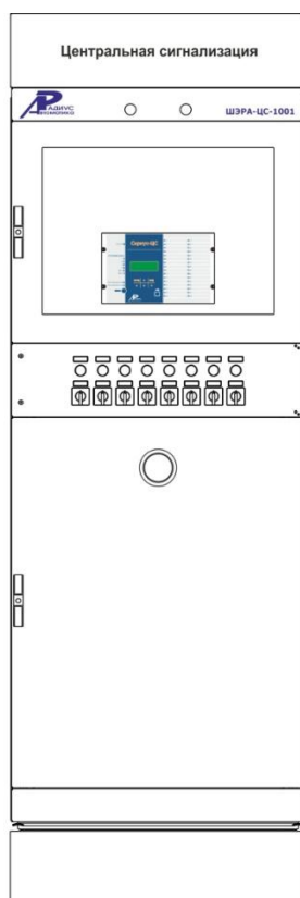
Шкаф центральной сигнализации ШЭРА-ЦС-1001 БПВА.656457.003, БПВА.650645.001 ТУ
