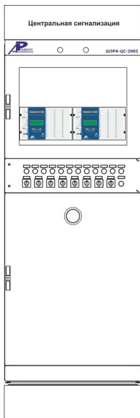
Шкаф центральной сигнализации ШЭРА-ЦС-2002 БПВА.656457.206, БПВА.650645.001 ТУ
