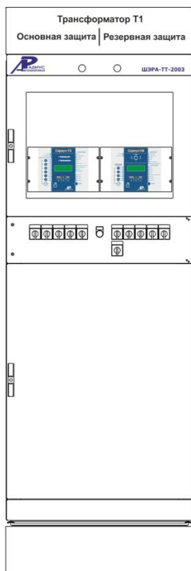
Шкаф защит трехобмоточного трансформатора и АУВ стороны ВН ШЭРА-ТТ-2003 (БПВА.656457.397, БПВА.650645.001 ТУ)
