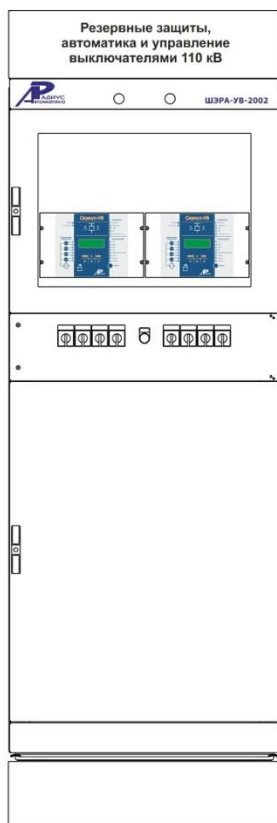
Шкаф резервных защит и АУВ двух присоединений 110(220) кВ ШЭРА-УВ-2002 БПВА.656457.500, БПВА.650645.001 ТУ
