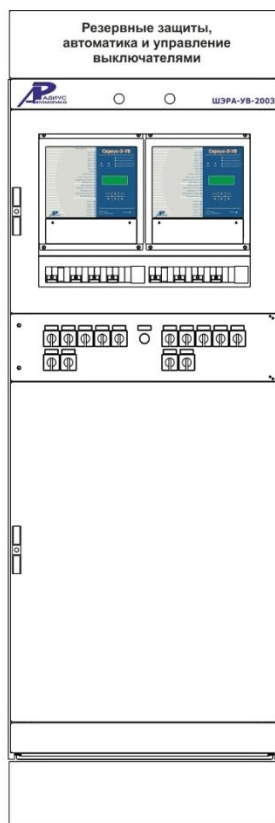
Шкаф резервных защит и АУВ двух присоединений 110(220) кВ ШЭРА-УВ-2003 БПВА.656457.505, БПВА.650645.001 ТУ
