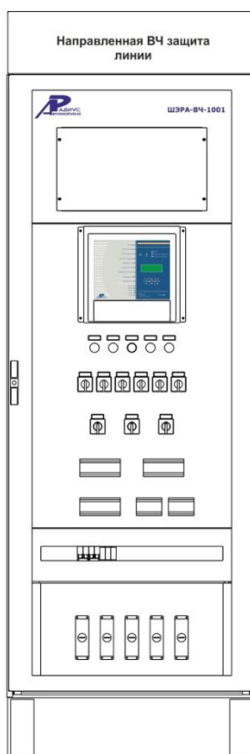
Шкаф направленной ВЧ защиты линии ШЭРА-ВЧ-1001 БПВА.656457.203, БПВА.650645.001 ТУ
